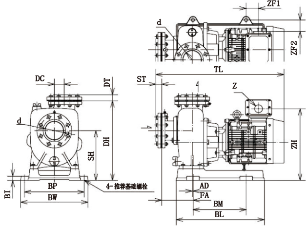
口径65-80场合
