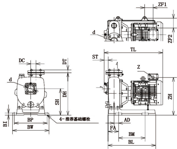
口径32-50场合
